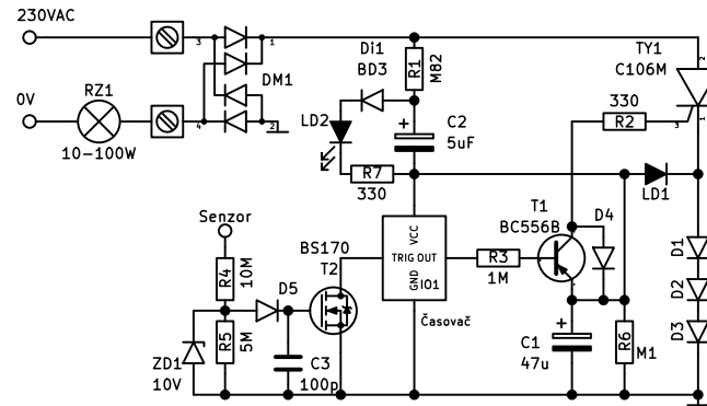
Kapacitní spínač 230V s časovačem GM.
